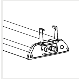
9905223 Sigma riputuskiskokannake 110
